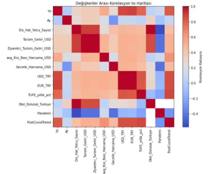
Şekil 10: Kolerasyon matrisi
